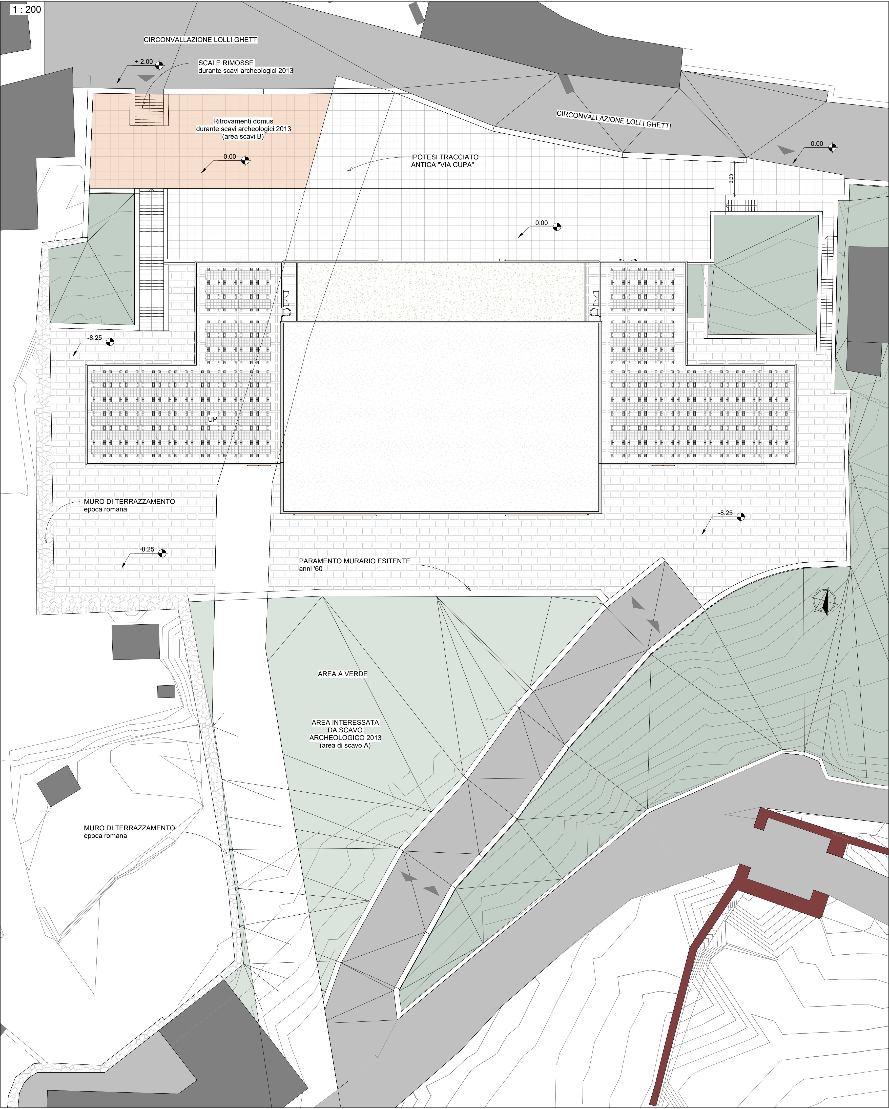
Pianta delle coperture
